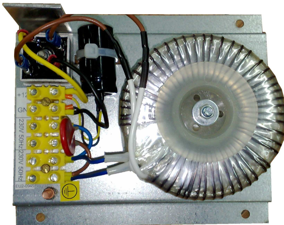
ZASILACZ SIECIOWY NIESTABILIZOWANY
