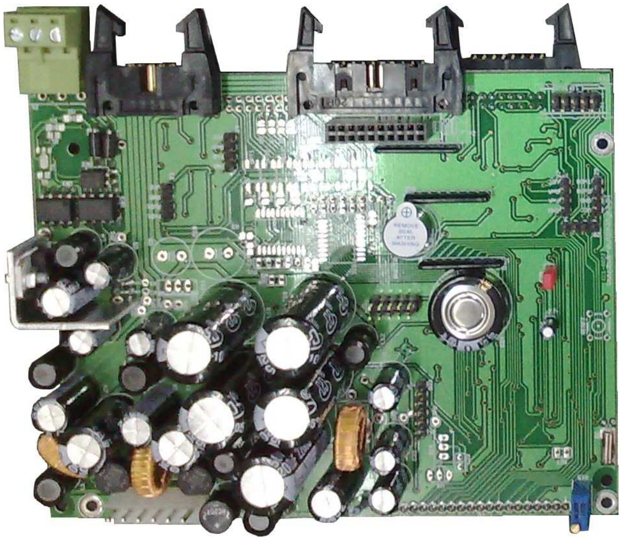
DEDYKOWANY UKŁAD STEROWANIA – WIDOK MONTAŻU THT
