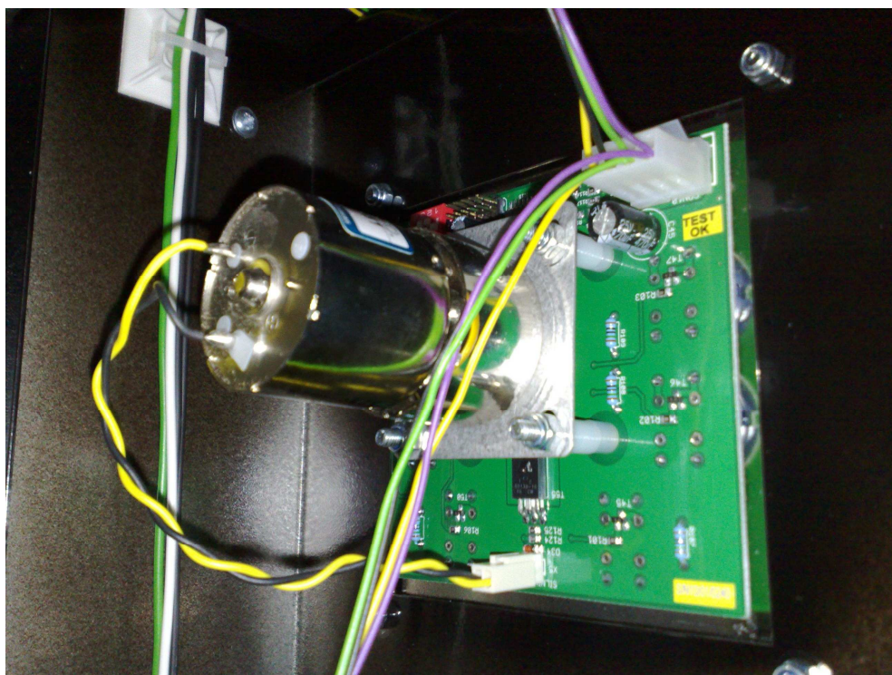
MODUŁ STEROWANIA SILNIKIEM PRĄDU STAŁEGO
