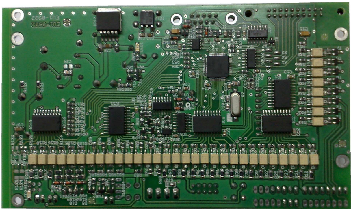
STEROWNIK DEDYKOWANY – MONTAŻ SMD
